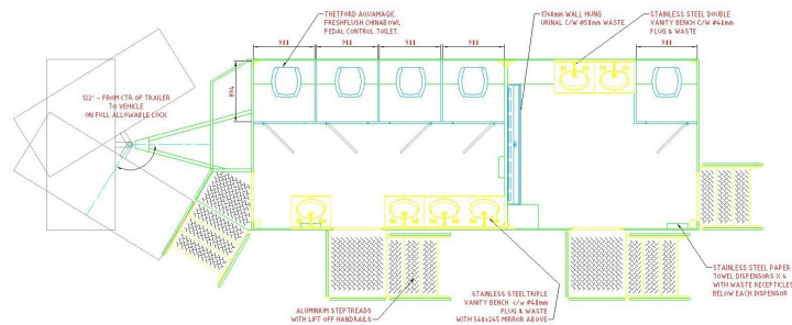
PLANVIEW OF TOILET
